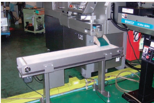
レイアウトに合せコンベアの向きが変更されます
